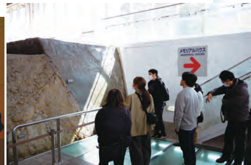
ずれた地層の様子
