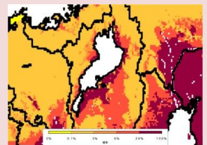
確率論的地震予測値図 濃色ほど高い発生率を示す
